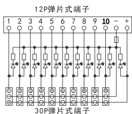
D1264-10P
