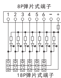
D1264-P
