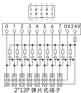
D1264-10P
