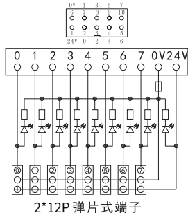
D1264-16
