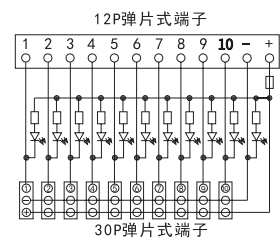
D1264-16P
