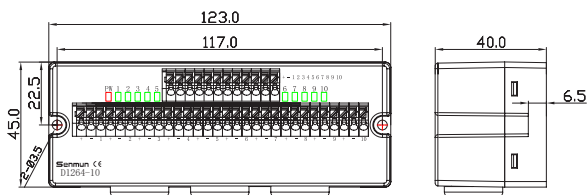
D1264-10/D1264-10P
