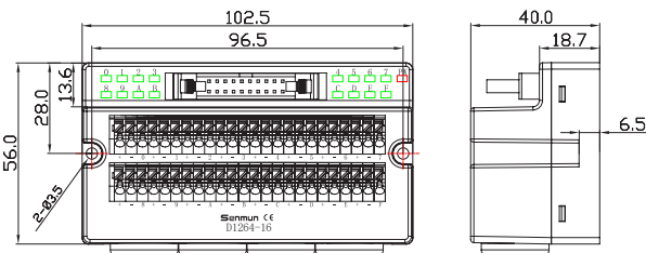
D1264-16/D1264-16P
