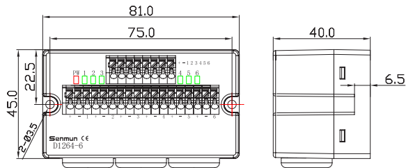
D1264-6/D1264-6P
