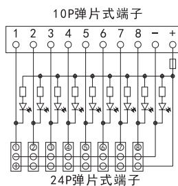
D1264
