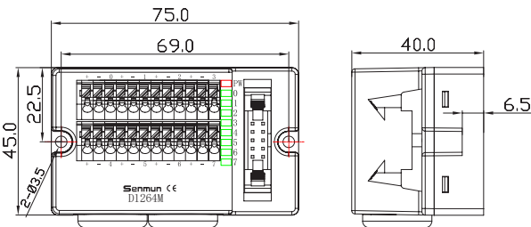
D1264M/D1264M-P
