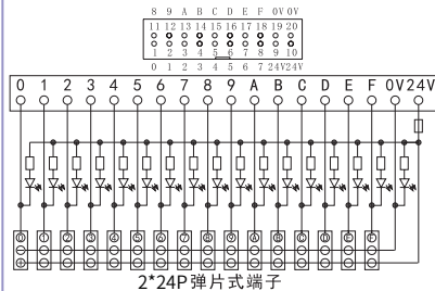
D1264-16
