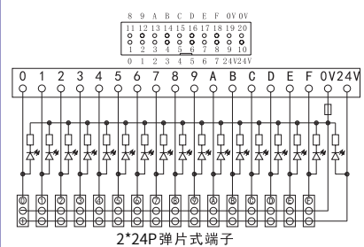
D1264-16P
