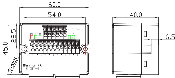
D1264/D1264-P
