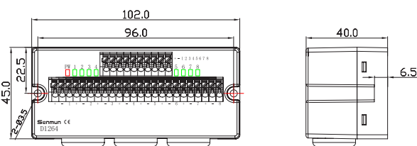
D1264/D1264-P
